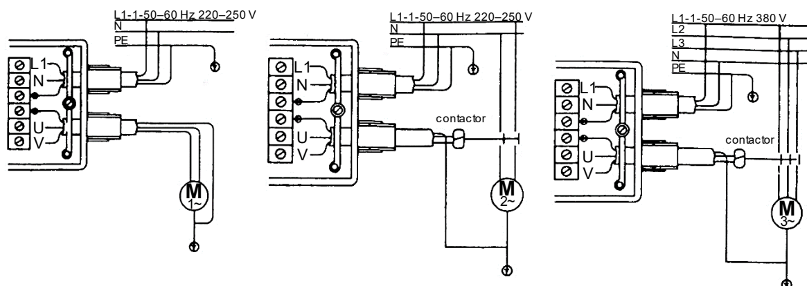
Aansluitschema voor eenfasige 220-V-pompen tot 1,1 kW
