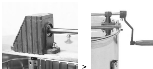
Bild 2: Fäst handvev.
