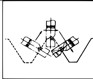
Seitenansicht – Der Stanzspan muss im rechten Winkel (90°) zur Oberfläche des zu schneidenden Werkstücks stehen.
