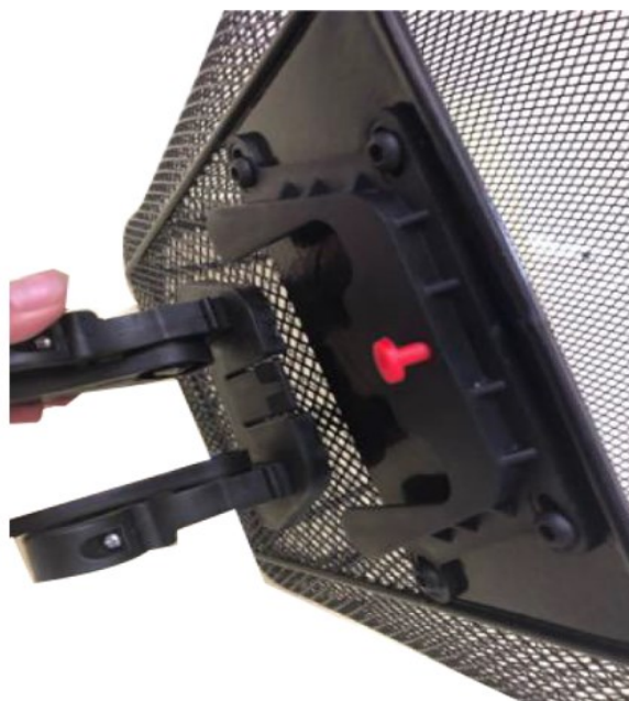
8. Druk nu de mand met de buitenste plaat tegen de houder. Druk de rode knop in en schuif de mand naar beneden totdat deze inklikt.
