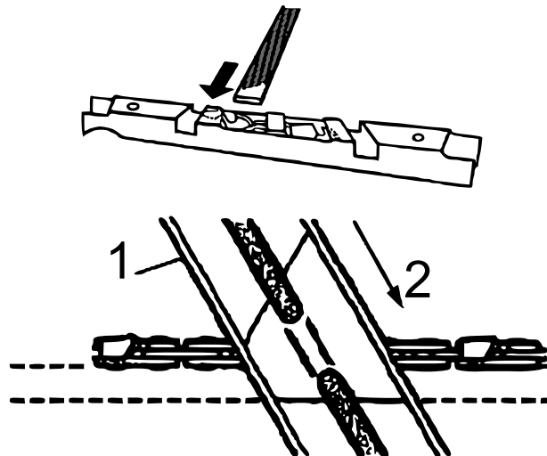
(1) Feilenhalterung; (2) Bewegungsrichtung
