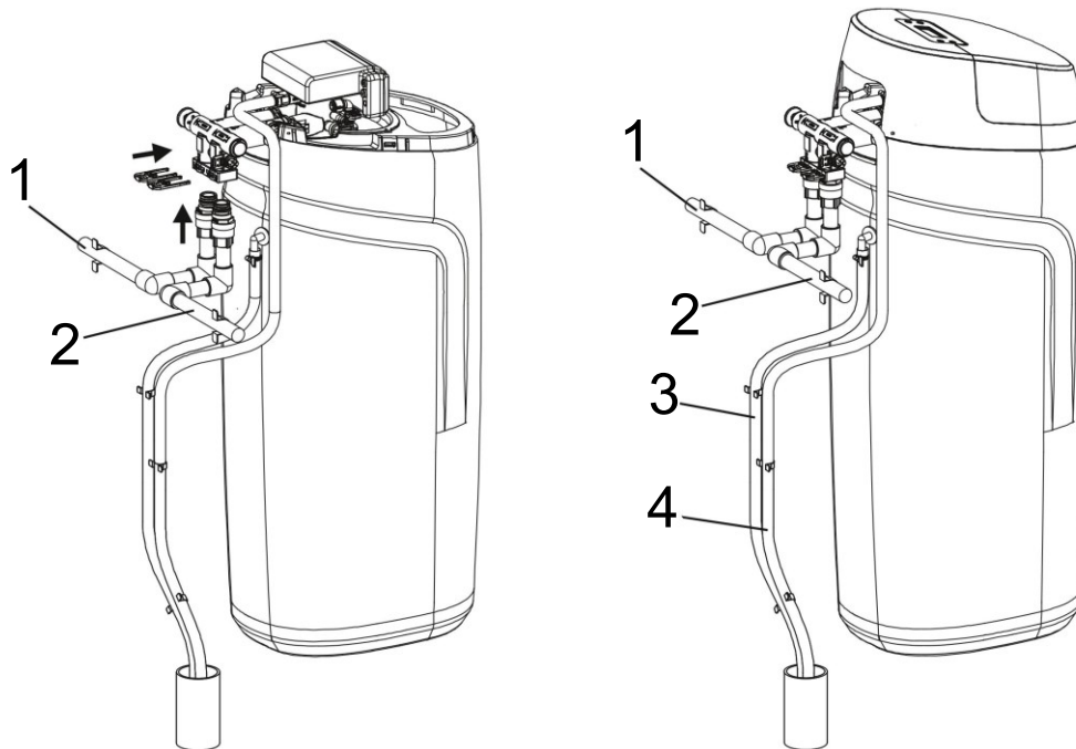
Schema di installazione dell'apertura di ingresso e uscita dell'acqua
